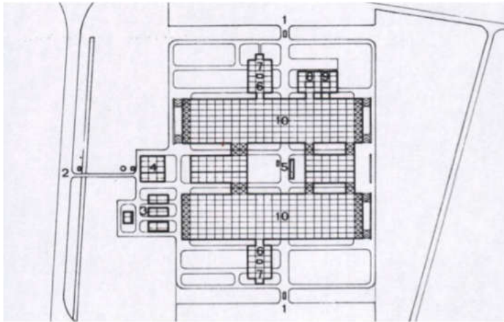
Planimetria del complesso di Marcinise.
